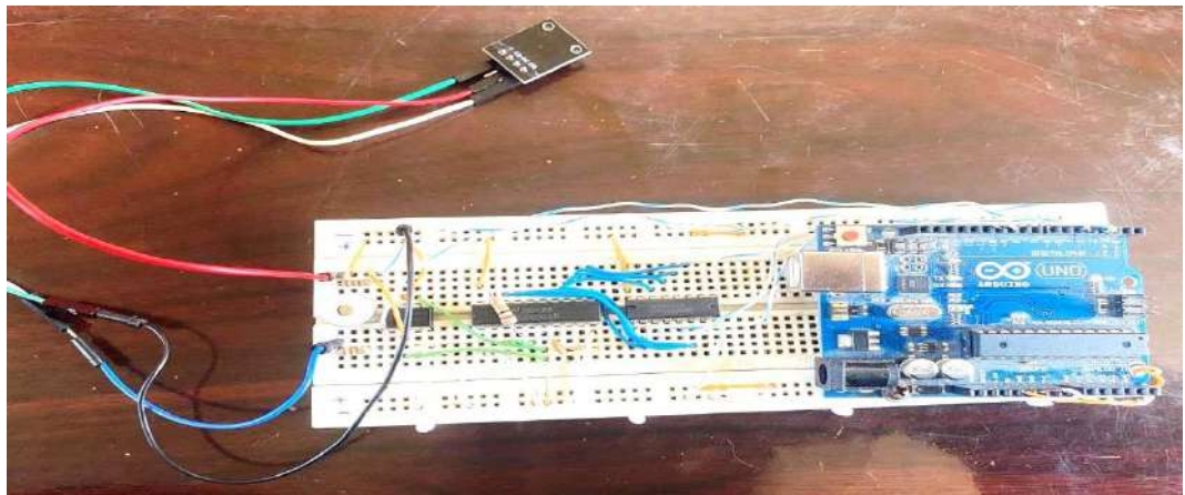
شكل رقم (10): دائرة إرسال Li-Fi باستخدام RGB LED.
